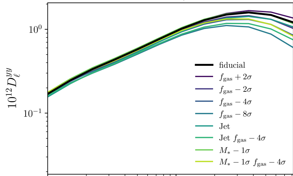
q > 10
