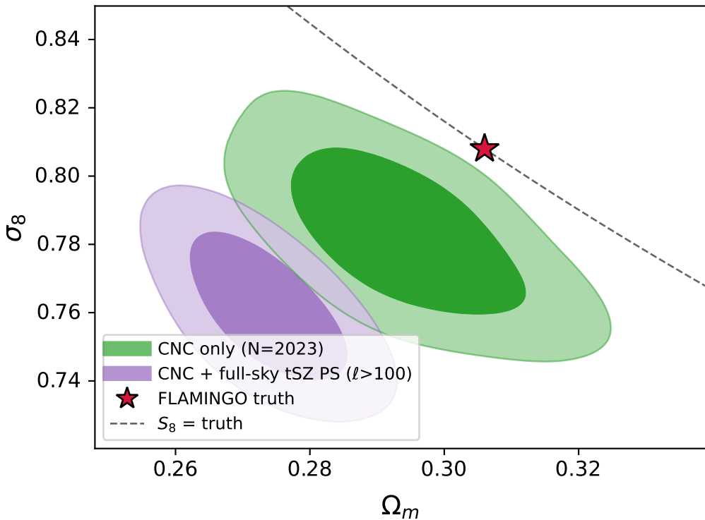
arnaudB1 Y_{R500c} : CNC vs CNC+tSZ PS
