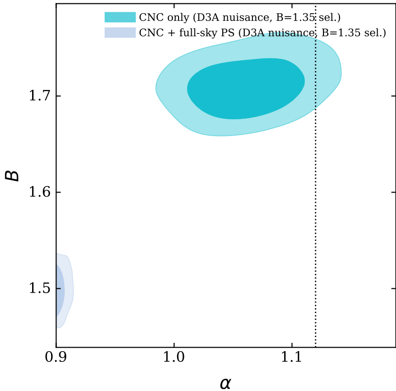
D3A nuisance, B=1.35 sel.: \alpha _SZ vs B
