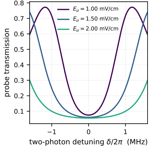
(d) conventional EIT-AT, same fields
