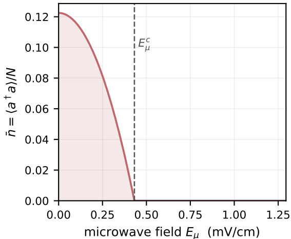
(b) order parameter at fixed \lambda
