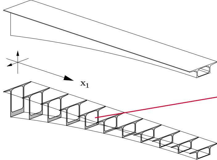
a) variação da seção
