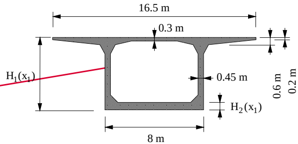
b) Seção transversal
