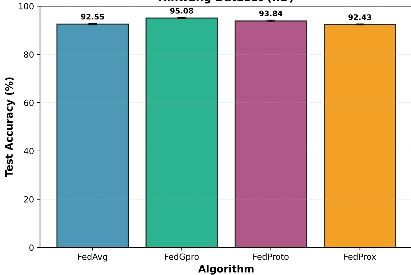
Xinwang Dataset (IID)
