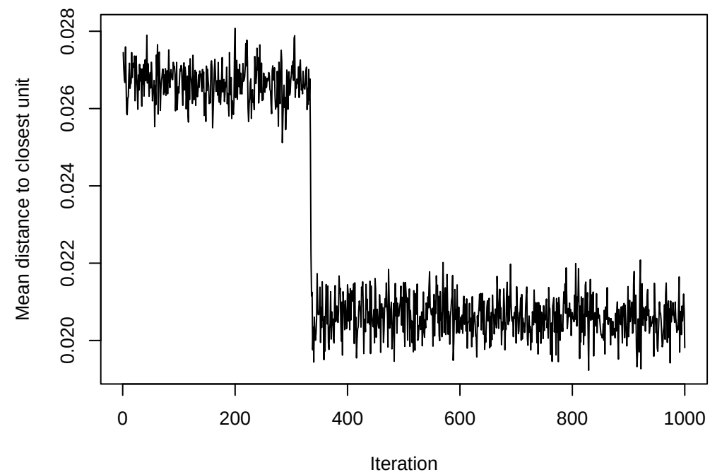
Convergencia do treinamento
