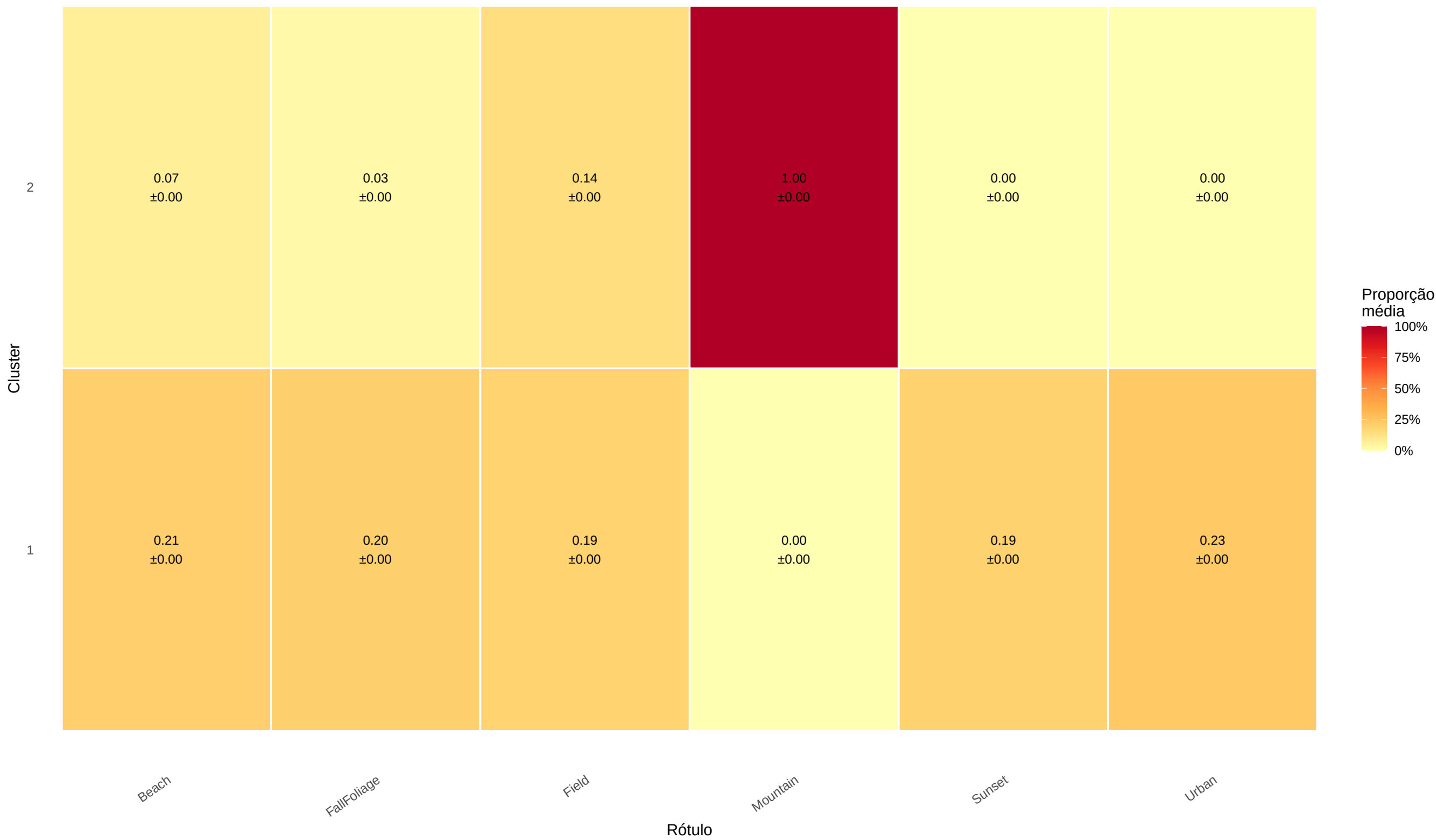
Heatmap de rótulos por cluster — scene | gaussian Células: proporção média (linha 1) ± DP entre folds (linha 2)
