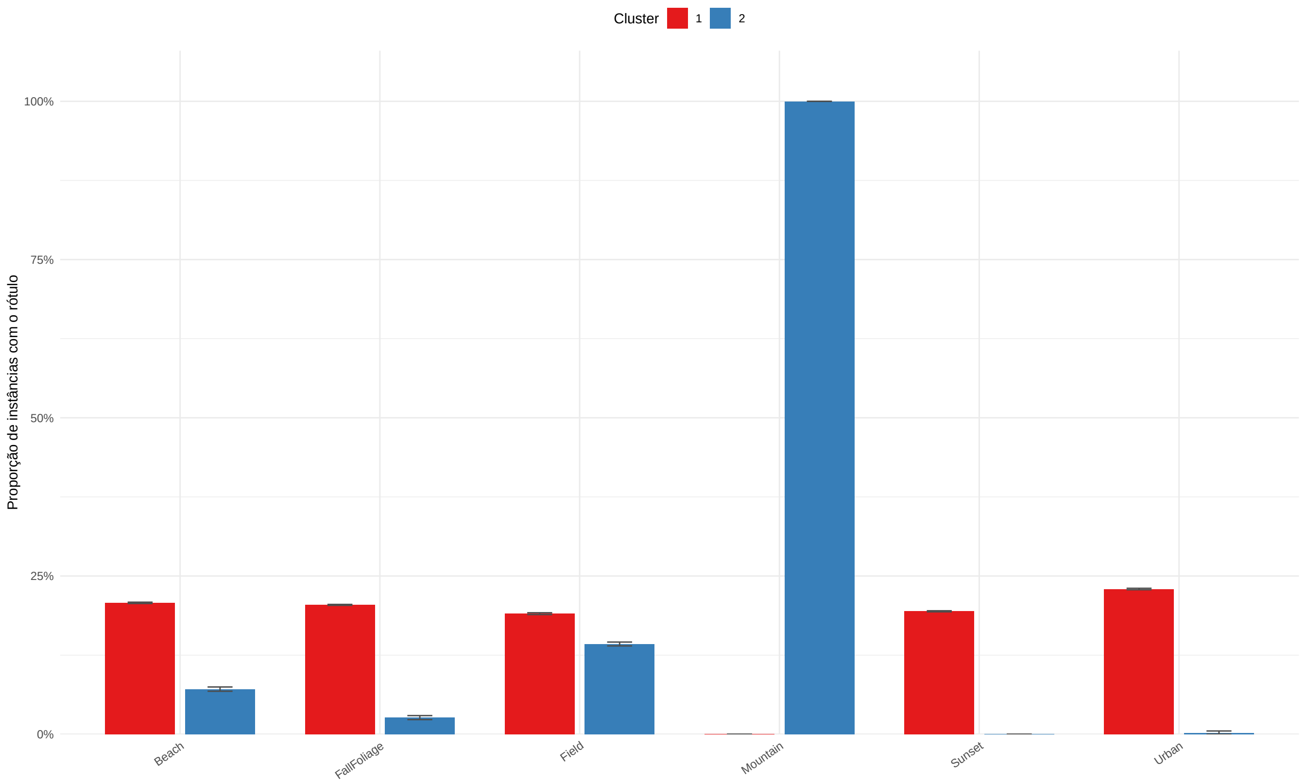
Proporção média de rótulos por cluster — scene | gaussian Barras de erro = \pm 1 DP entre folds · quanto mais sobrepostas, mais instável a partição
