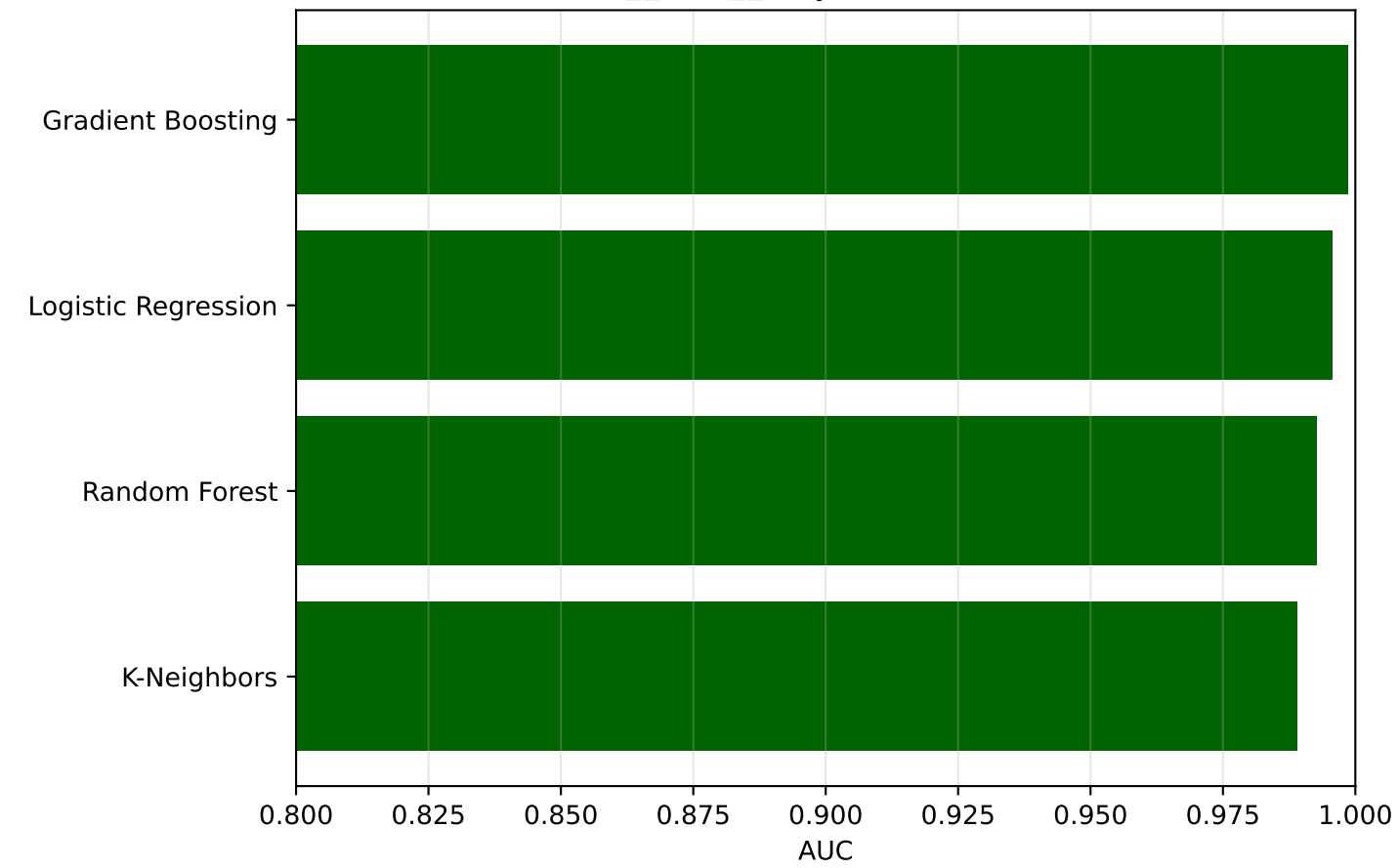
AUC - Python/sklearn
