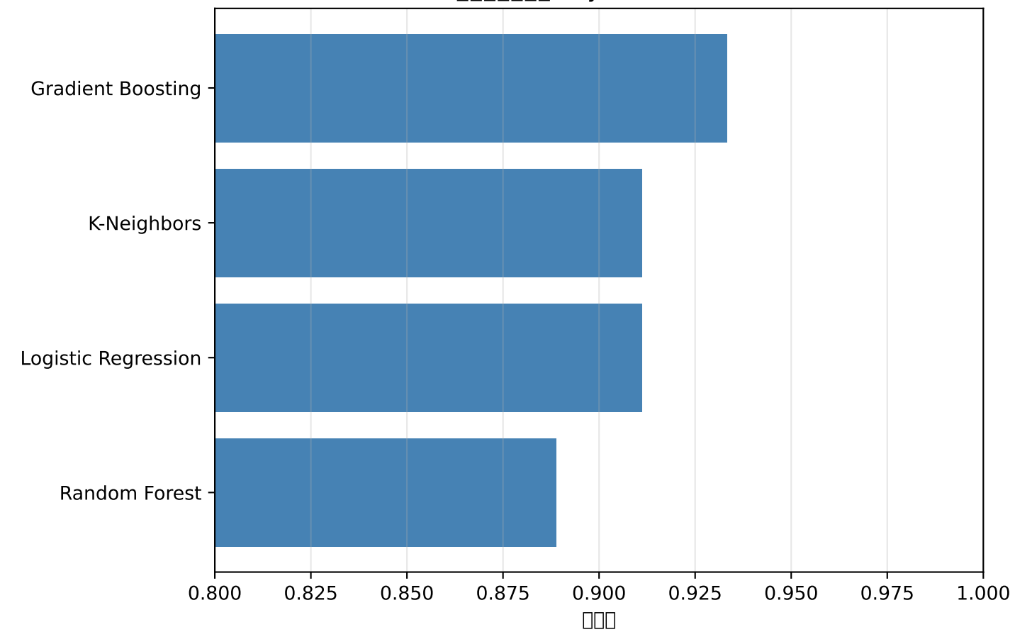
AUC - Python/sklearn
