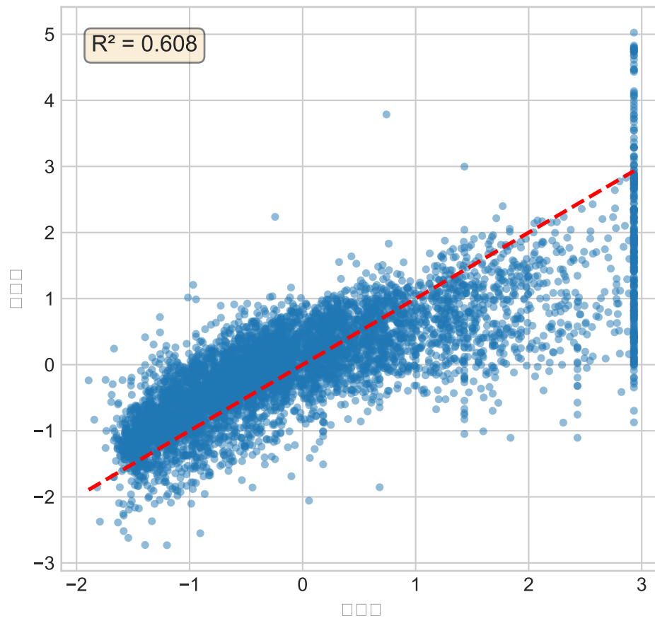
Lasso: y vs x
