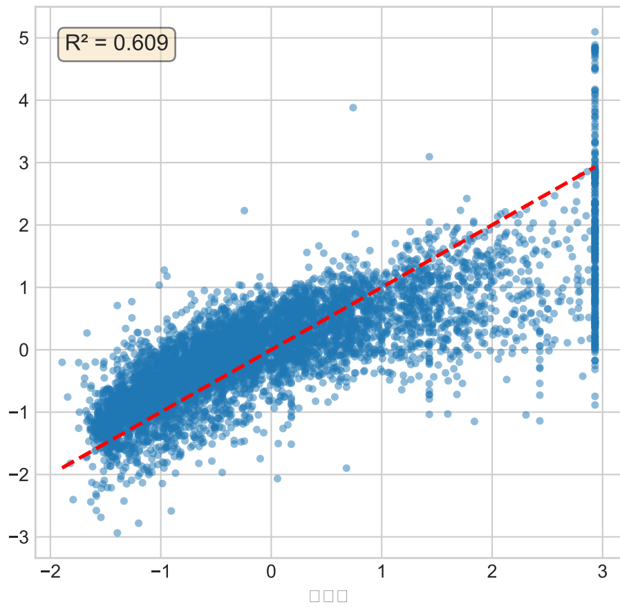
OLS: y vs x
