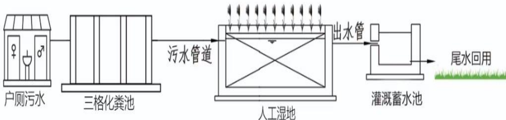
农村分户式“四件套”设施工艺流程示意图
