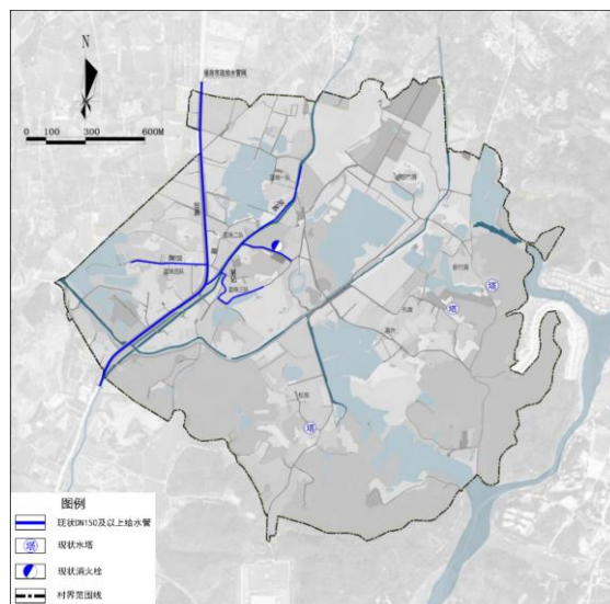
竹洞村给水工程现状图
