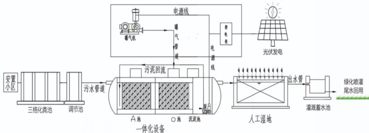
农村一体式微动力污水处理设施工艺流程示意图
