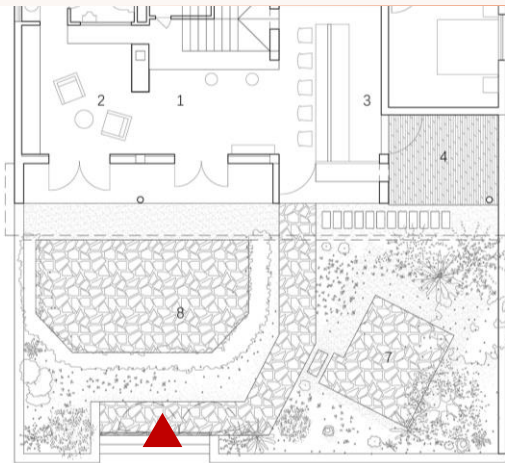
庭院入口 一层平面
