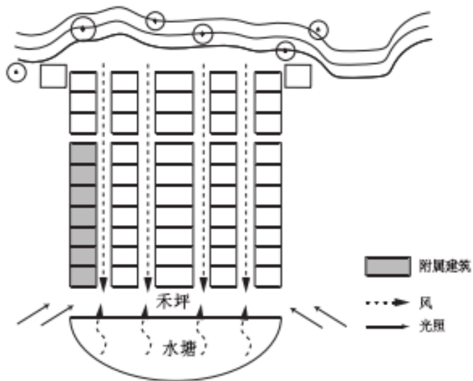
在炎热潮湿地区产生的梳式布局
