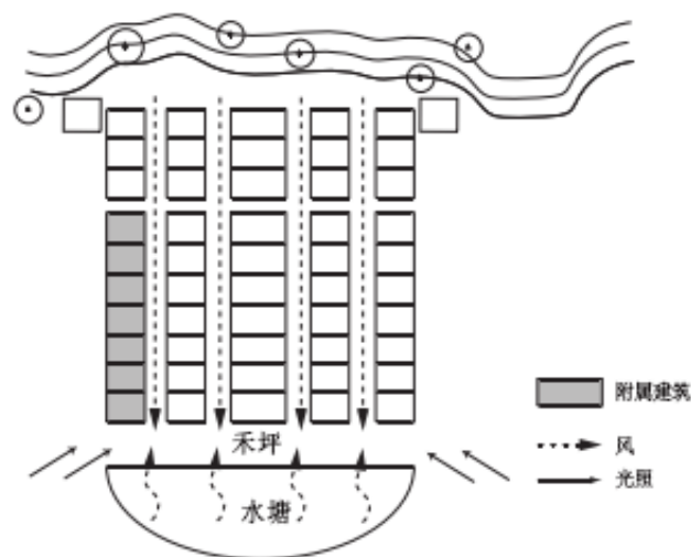
梳式布局原型
