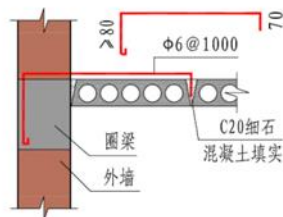
预制板侧面与外墙拉结(✓)
