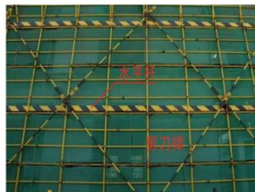
设置横杆、剪刀撑 (✓)
