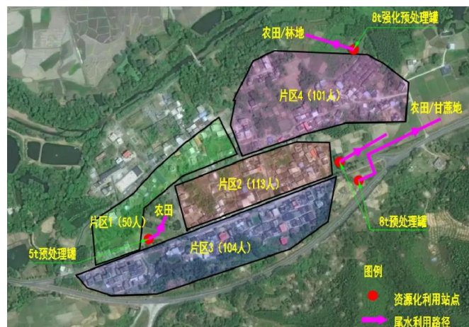
珍珠村联户污水治理模式图
