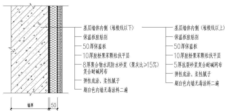
外墙内保温系统做法 (一)
