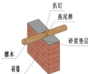
相邻檩木采用燕尾榫、扒钉连接(✓)
