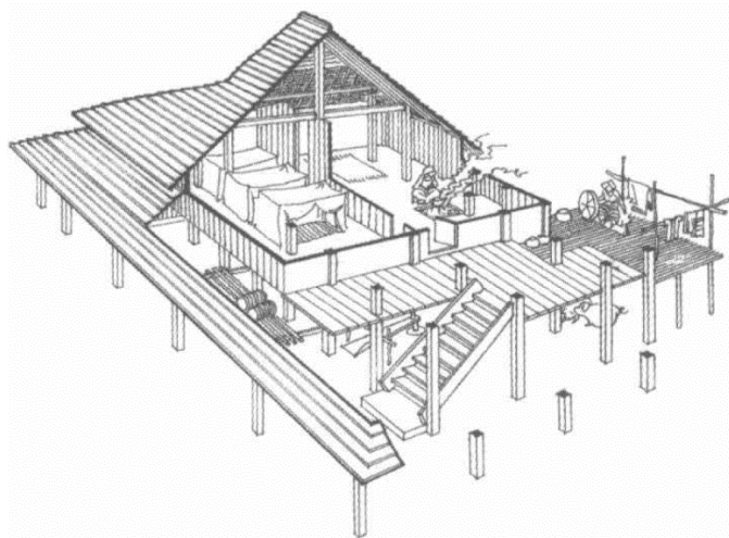
图 傣族竹楼剖透图
