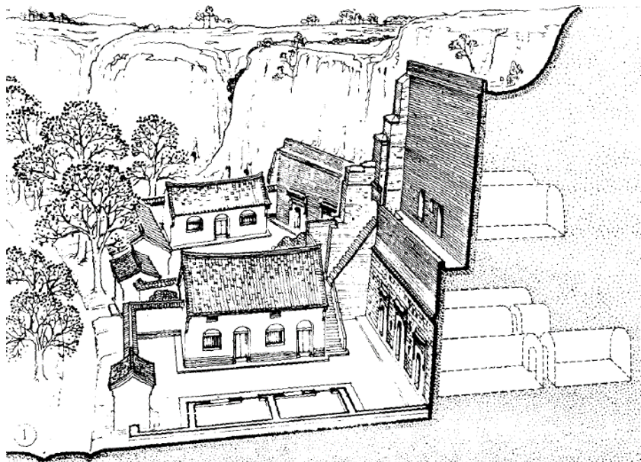
图 靠崖窑
