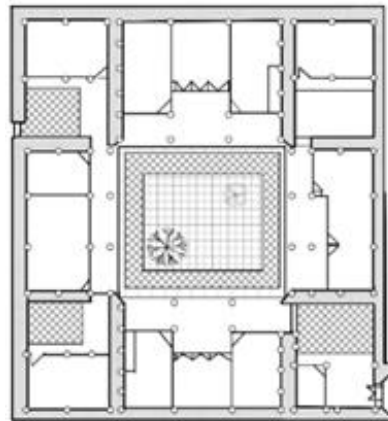
图 大理白族一颗印平面图
