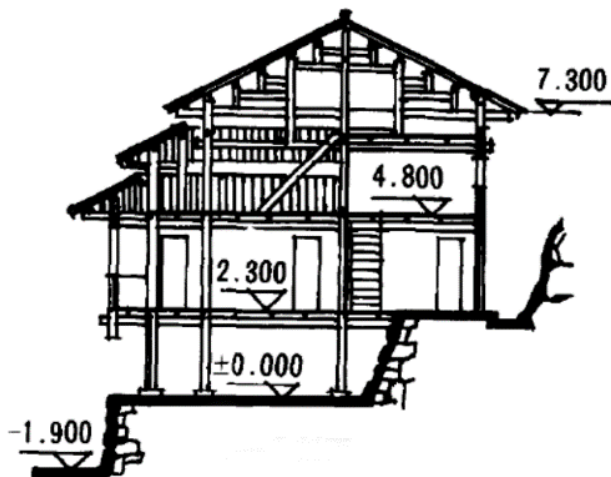
图 侗族干栏式建筑剖面
