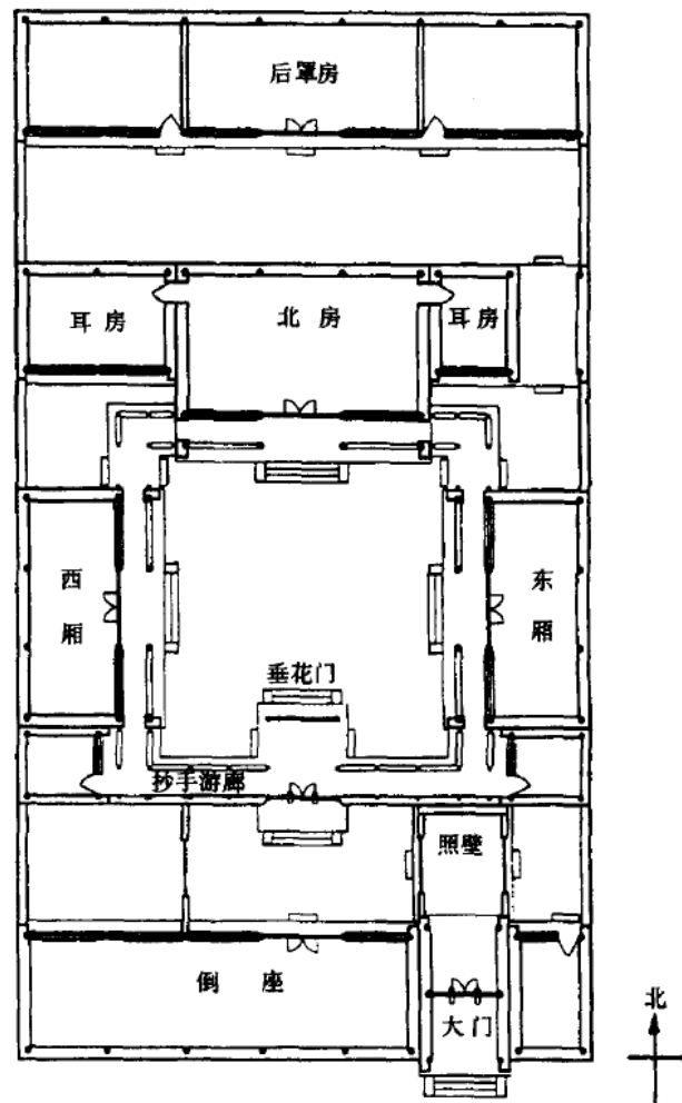
图 标准三进四合院平面图
