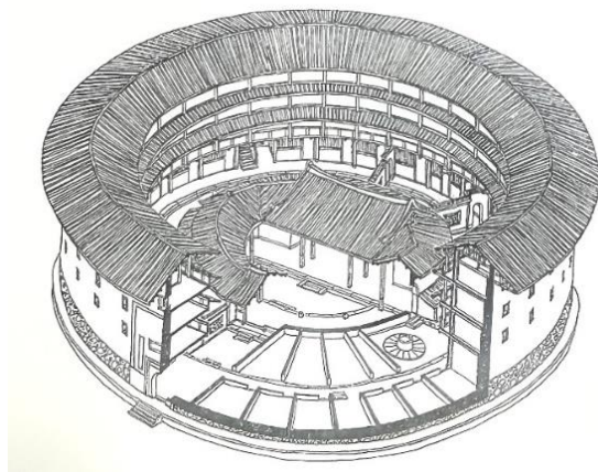
图 圆楼-福建南靖梅林怀远楼
