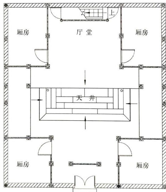
图 “四水归堂”——徽州民居平面
