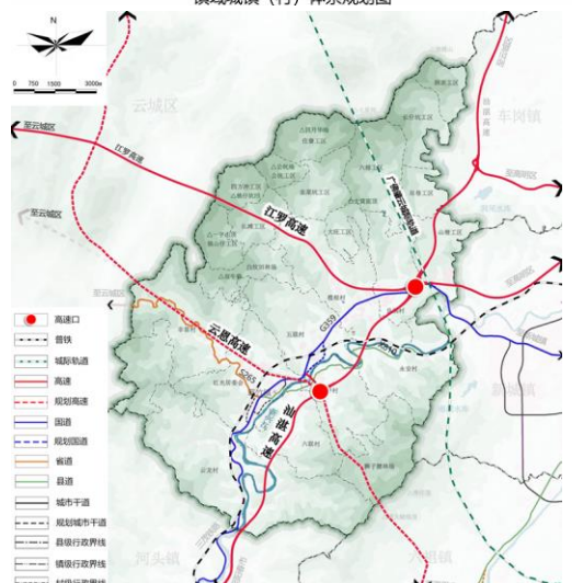
镇域综合交通规划图
