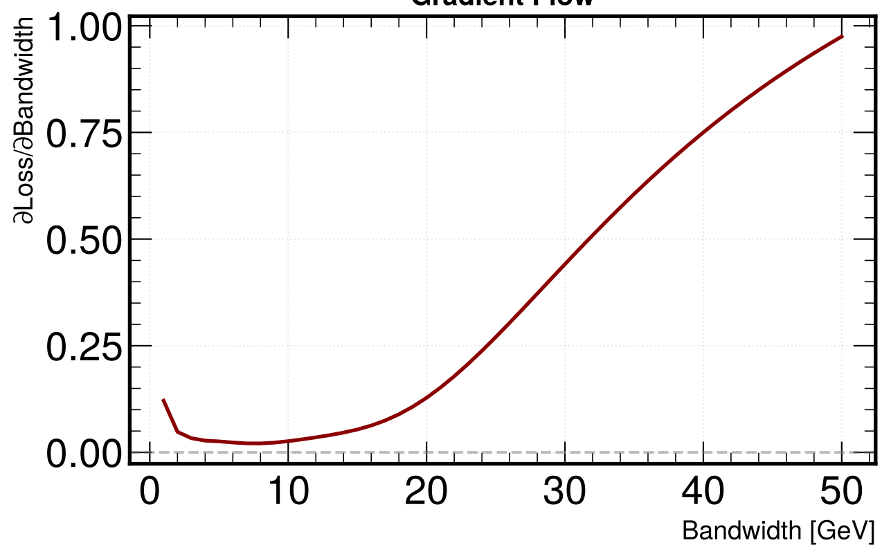
Gradient Flow
