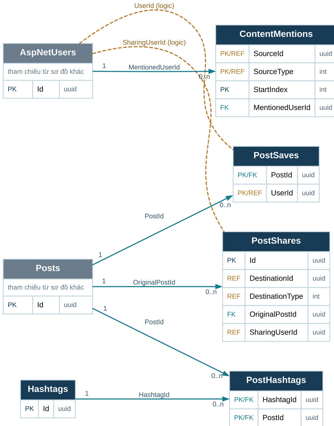
Hình 06. 06-social-interactions.svg — bản SVG trong docs/erd cho phép phóng to.
