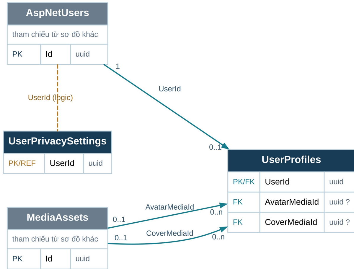
Hình 03. 03-users.svg — bản SVG trong docs/erd cho phép phóng to.
