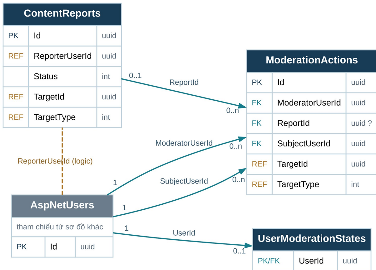
Hình 13. 13-moderation.svg — bản SVG trong docs/erd cho phép phóng to.
