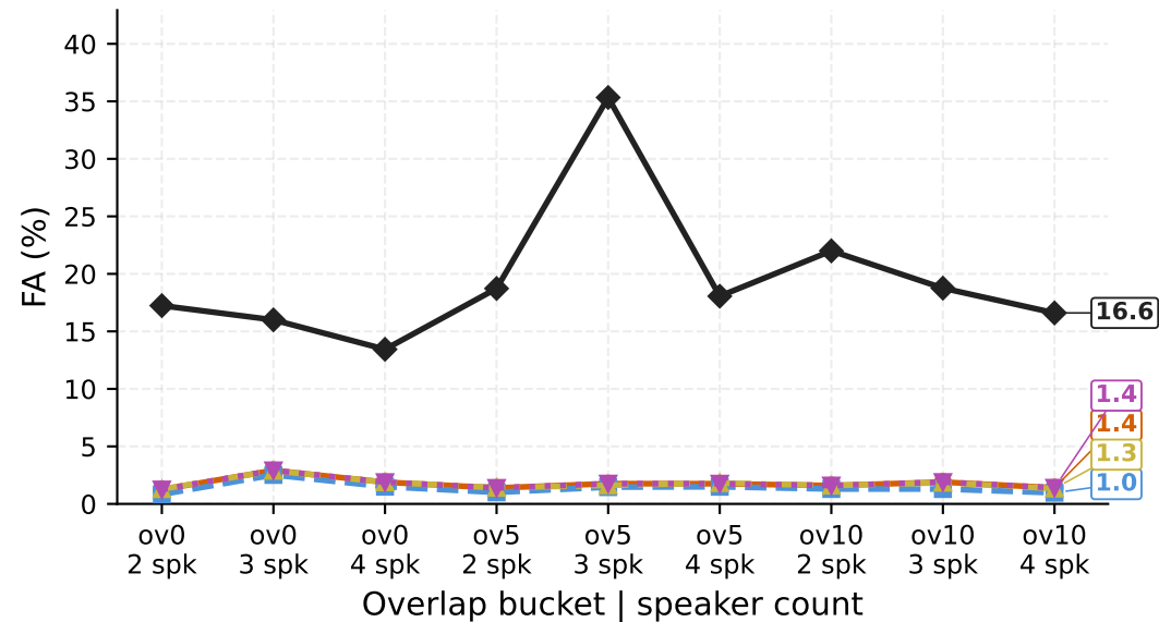
FA (%)
