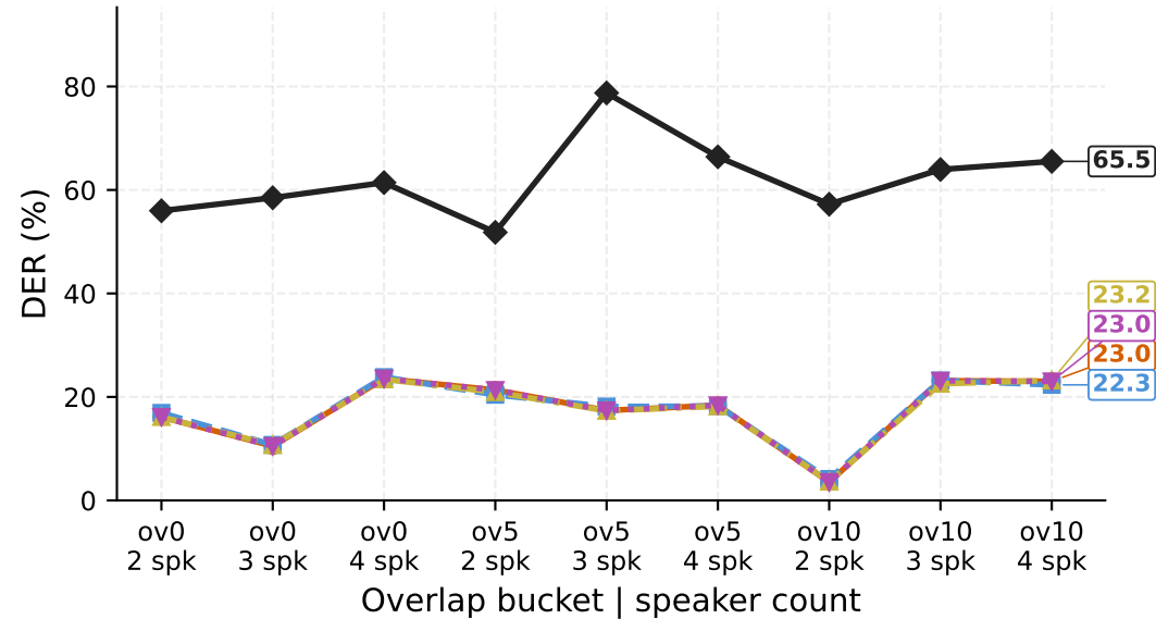
DER (%)
