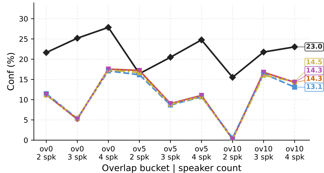
Conf (%)
