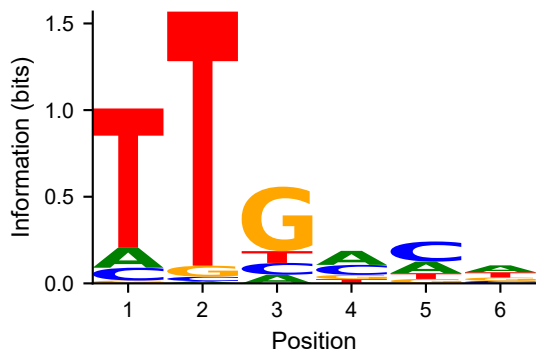
Best -35/-10 spacer distribution
