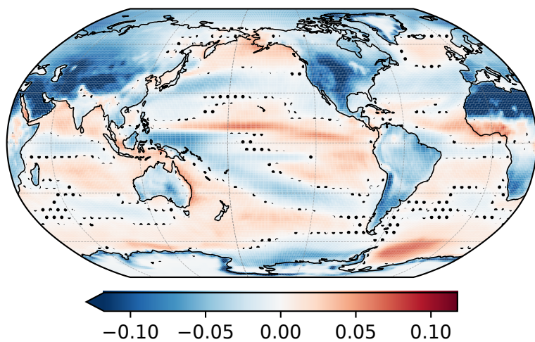
(d) Shortwave — TOA
