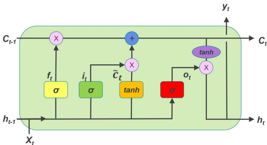
图 5.4 LSTM 结构图
