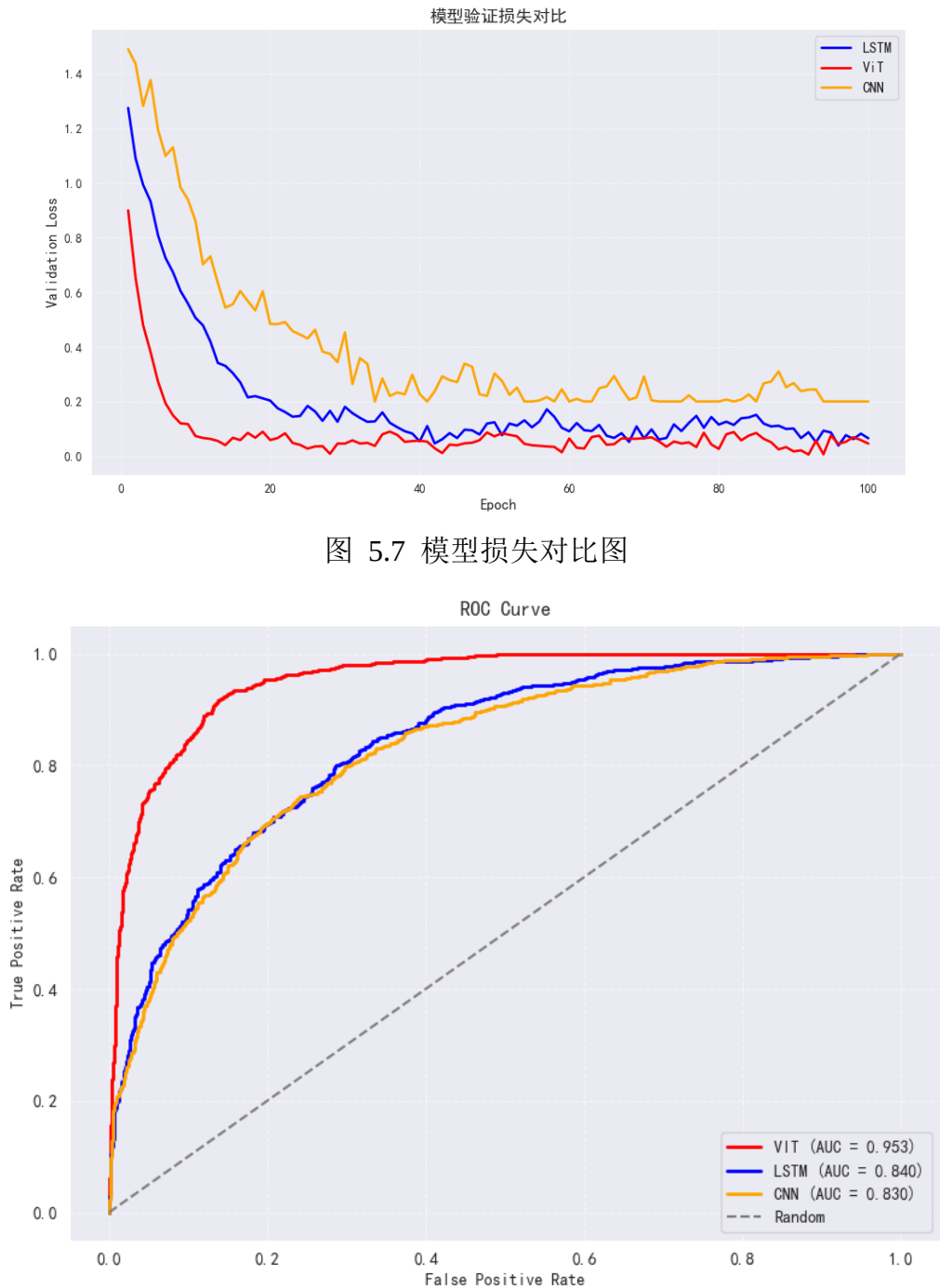
图 5.8 ROC 对比图
