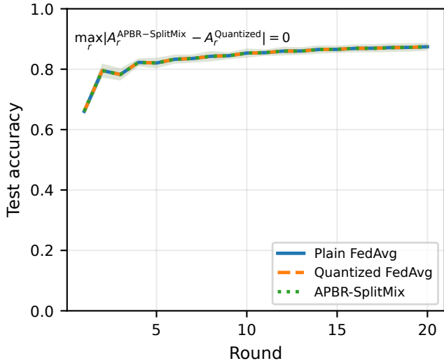
MNIST
