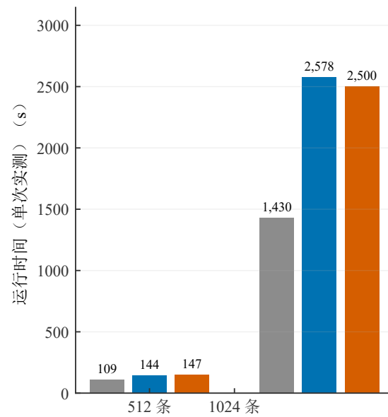
运行时间（单次实测）
