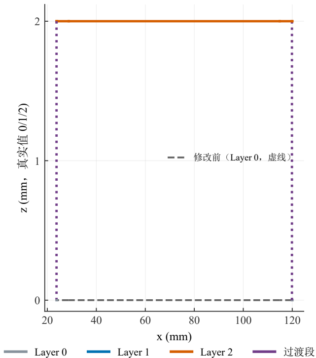
XZ 侧视 (沿程高度)
