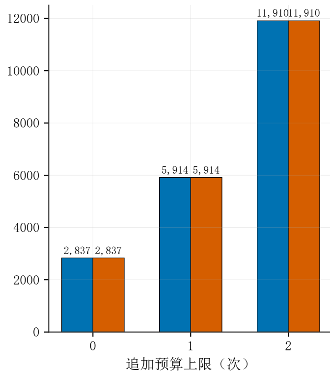
(b) 相对起点减少对数
