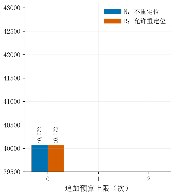
(a) 终态近距对数
