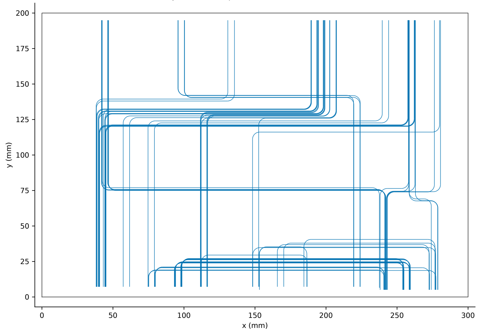
Layer 1: actual planar sections at z = 1\text{ mm}
