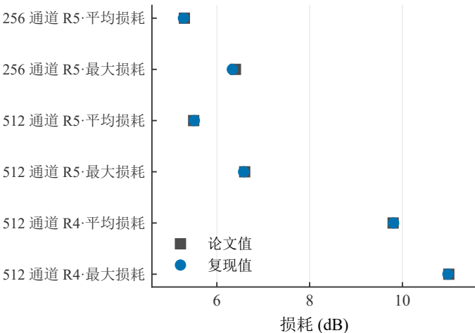
(a) 论文值与复现值（连线为同一指标）
