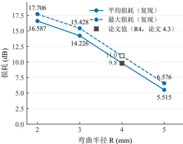
(a) 512 通道半径扫描 (离散半径 2/3/4/5 mm)
