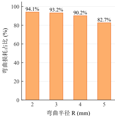
(b) 弯曲在总损耗中的占比
