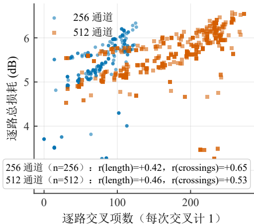
(b) 损耗 vs 交叉数
