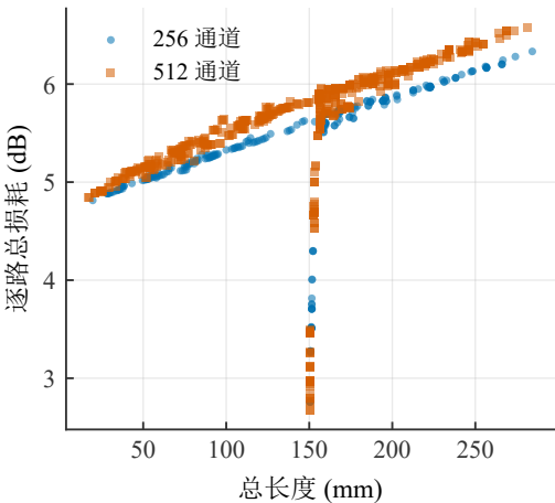
(a) 损耗 vs 总长度
