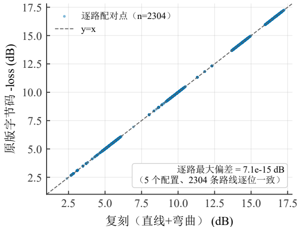
(b) 逐路对照 (原版 Python 3.8 字节码实跑)
