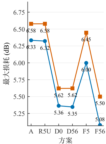
(c) 最大损耗
