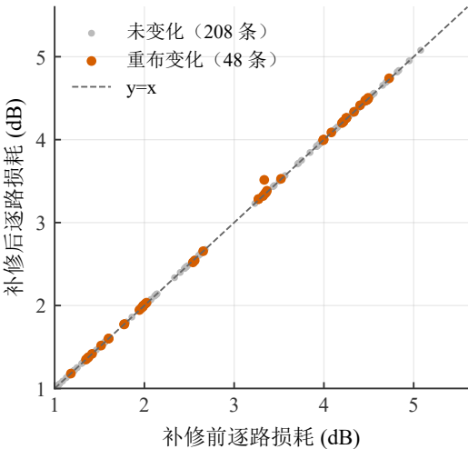
(a) 256 通道 F56 补修前后逐路对照
