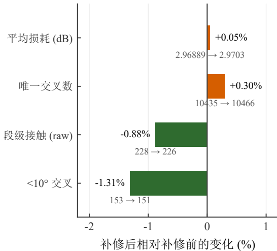
(b) 256 通道 F56 补修前后变化率 (#7/#31 重合 152.007 mm)
