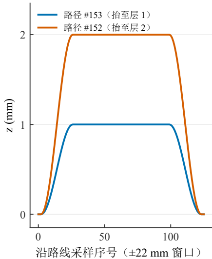
(b) 抬层示例侧视
