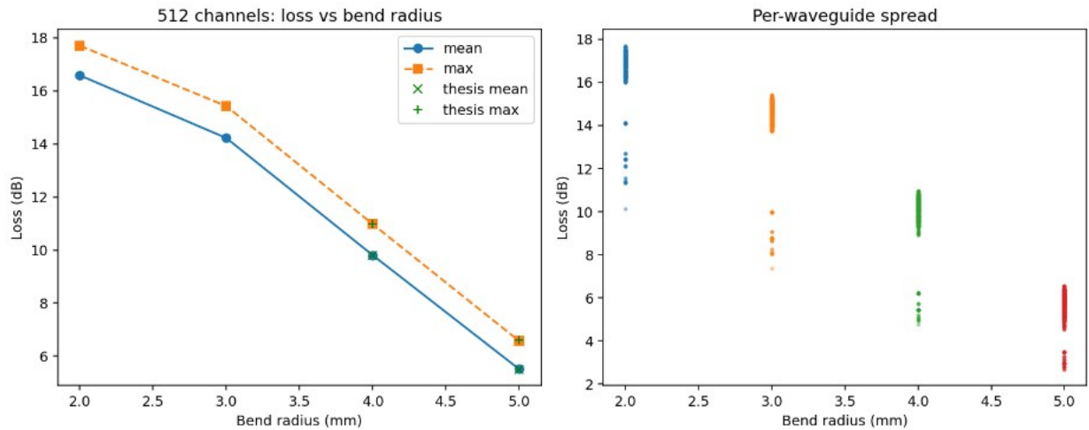
图 2 自己的半径扫描结果 左为损耗汇总 右为逐条路线分布
