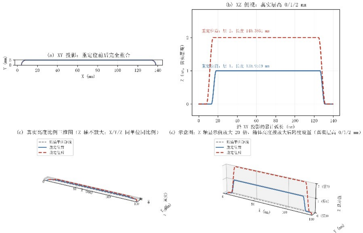
图 12 自己的结果：路线 34 被接受的这一次重定位前后（XY 投影、XZ 侧视、真实高度比例三维图、Z 轴放大 20 倍示意图；真实层高 0/1/2 mm）
