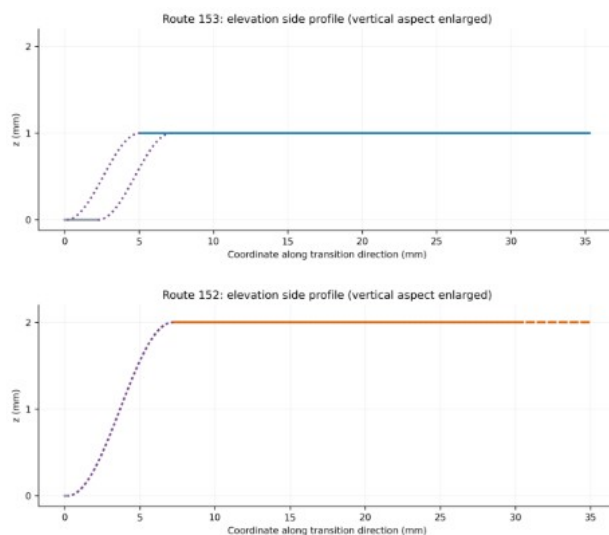
图 6 自己的局部抬层示例 左为 1 mm 层 右为 2 mm 层
