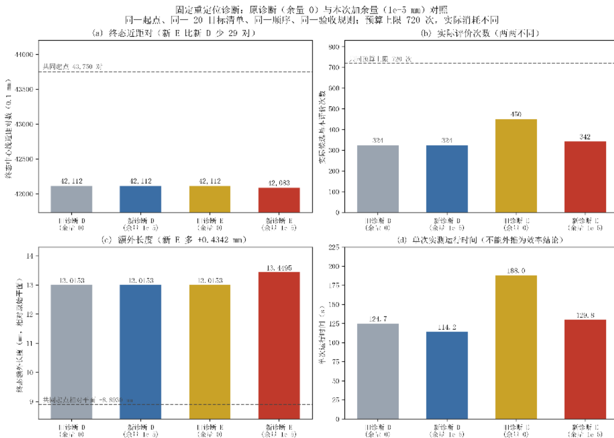
图 10 自己的结果：旧诊断（余量 0）与加余量诊断（ 1e-5 mm）的终态、实际评价次数、额外长度与单次运行时间对照
