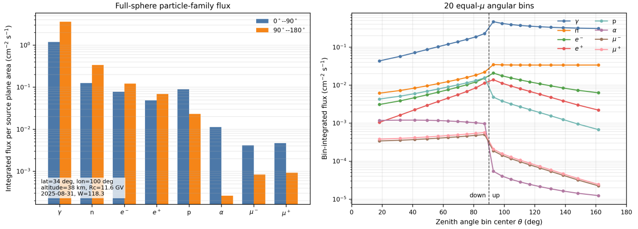
图 3: 用于生成瞬发和活化产生输运输入的 EXPACS/PARMA 全空间大气通量场。左: 八类运输粒子族的能量和立体角积分通量, 并按下行、上行半球分开。右: MEGALib 远场源使用的 20 个等 \mu 微分天顶角分箱的积分通量。该图直接由源定义输入表生成, 环境参数为纬度 34^\circ 、经度 100^\circ 、海拔 38\text{ km} 、 R_c = 11.6\text{ GV} 、 W = 118.3 。
