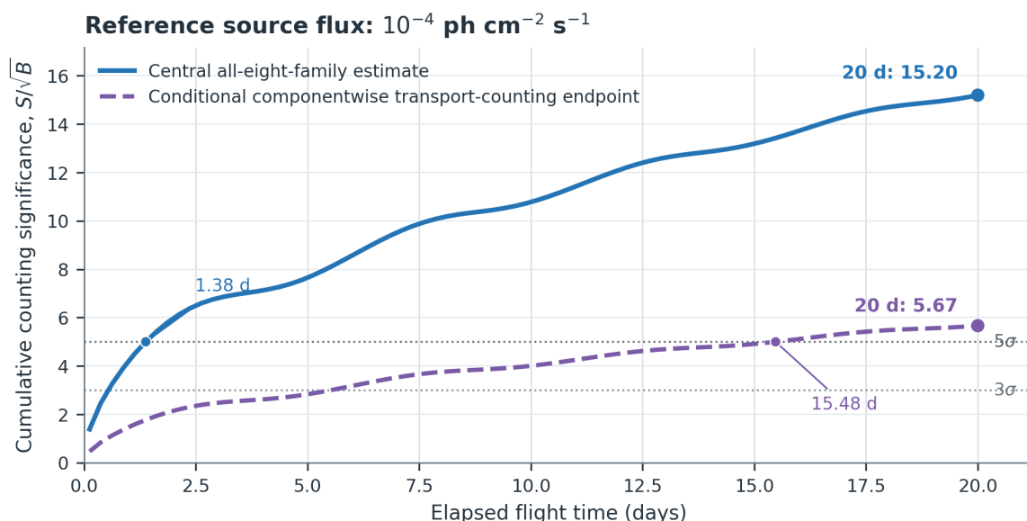
图 10: 最终方向分级屏蔽几何沿固定 45^\circ 仰角的 20 d 参考轨迹连续观测大气层顶 10^{-4} \text{ ph cm}^{-2} \text{ s}^{-1} 点源时的累计计数显著度。实线使用能量响应卷积后的中心选后率；虚线对每个本底分量使用精确 95% 计数上端，并对信号接受度使用精确 95% 下端。其逐分量组合是条件式端点，不是联合 95% 区间。两条曲线分别在 1.38 和 15.48 d 达到 5\sigma ，20 d 时分别达到 15.20 和 5.67。
