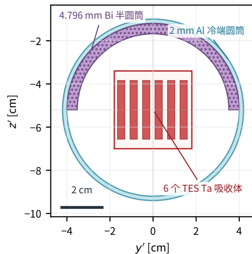
c Bi 半圆筒与六单元 TES 横截面
