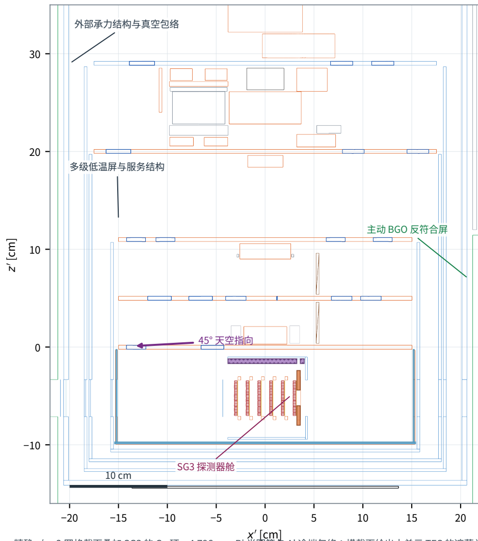
a SG3 探测器—低温系统完整质量模型
