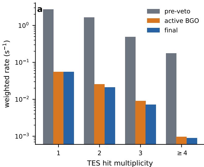
480--550 keV band
