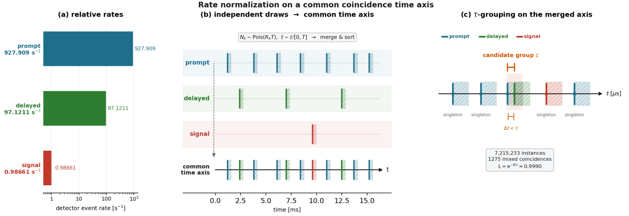
图 4: 率归一示意。(a) 全能段探测器事例率 (928、97.1、0.987 s -1 )。 (b) 三条流独立泊松抽样后合并排序到公共时间轴；颜色标识流身份，影线表示各事例的时间足迹。(c) \Delta t \leq \tau = 1 \mu\text{s} 的事例归为一个符合候选组；框内为参考曝光的偶然符合记账。事例位置为示意。
