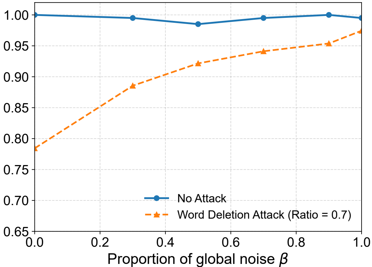
Detection F1 Score
