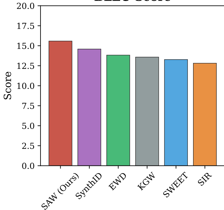
BLEU Score
