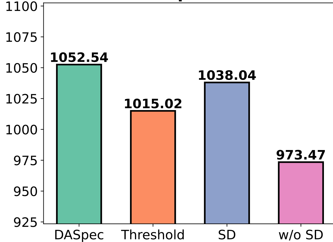
Alpaca
