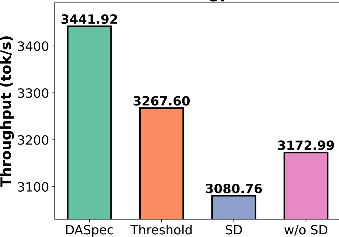
Sharegpt
