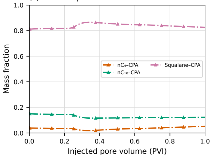
(d) Four-component CPA: HC-normalized
