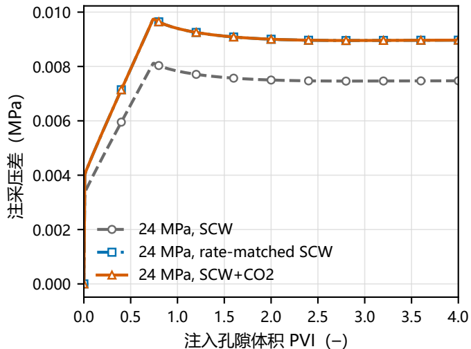
24 MPa
