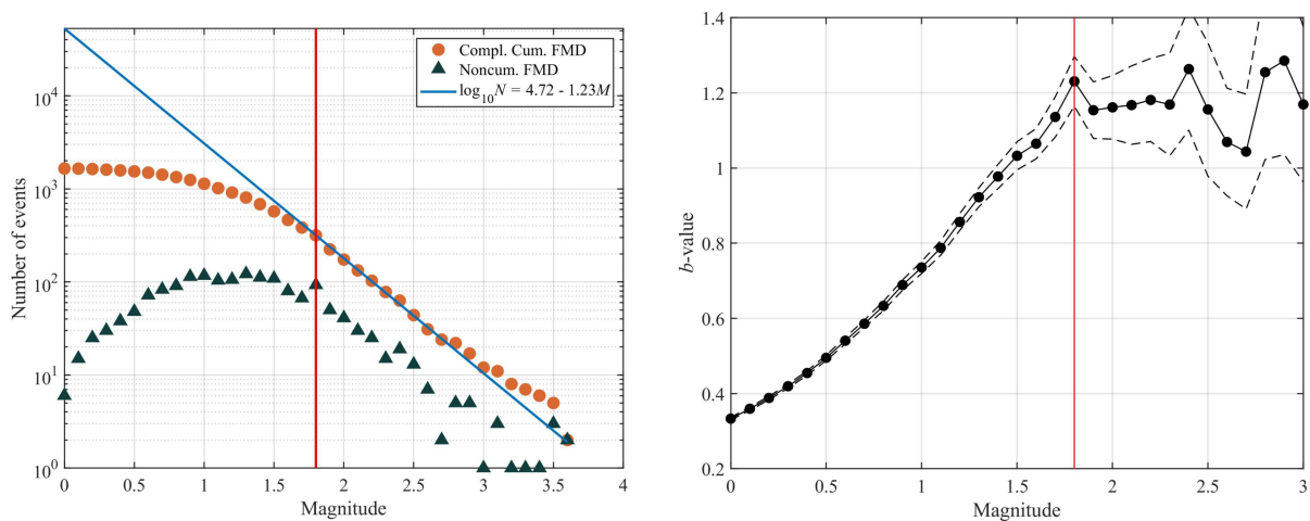
图 5. 过去一个月中国地震科学实验场地震活动性的（左）互补累积和密度震级-频次分布以及大于目录截止震级 M_{co} （红线）地震的古登堡-里克特（GR）关系拟合结果；（右） b 值随 M_{co} 变化的曲线，其中细虚线表示 \pm 1\sigma 的标准差。
