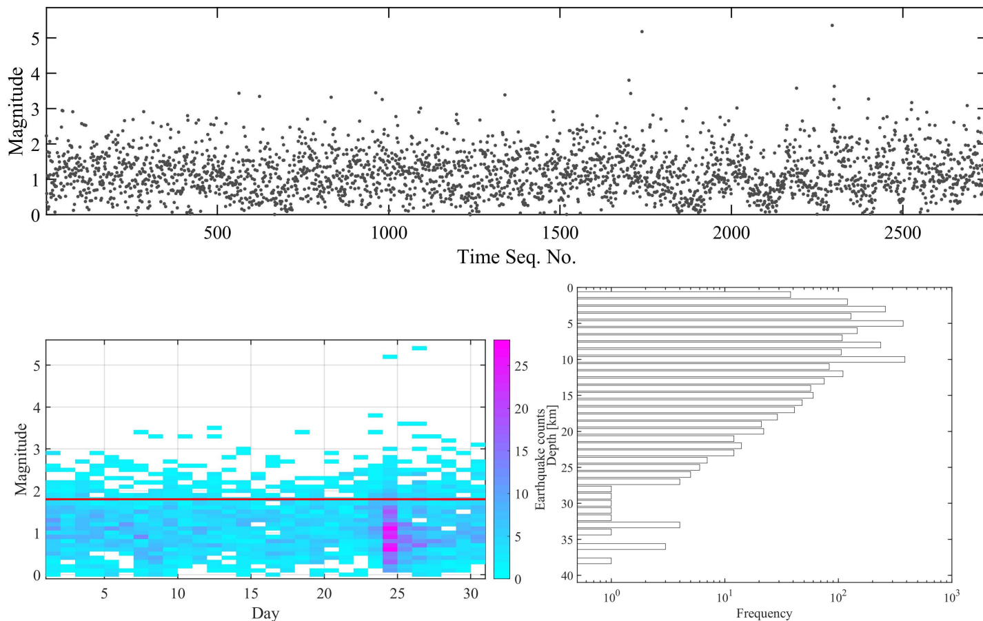
图 4. 过去一个月中国地震科学实验场地震活动性的 (上) 震级-时间序号图; (左下) 每 0.1 个震级区间的每日地震数量; (右下) 深度-频次分布。震级-时间序号图中的震级被添加了 [-0.05, 0.05] 均匀分布的随机误差。左下图中的红色直线为过去一个月的目录最小完整性震级 ( M_c )。
