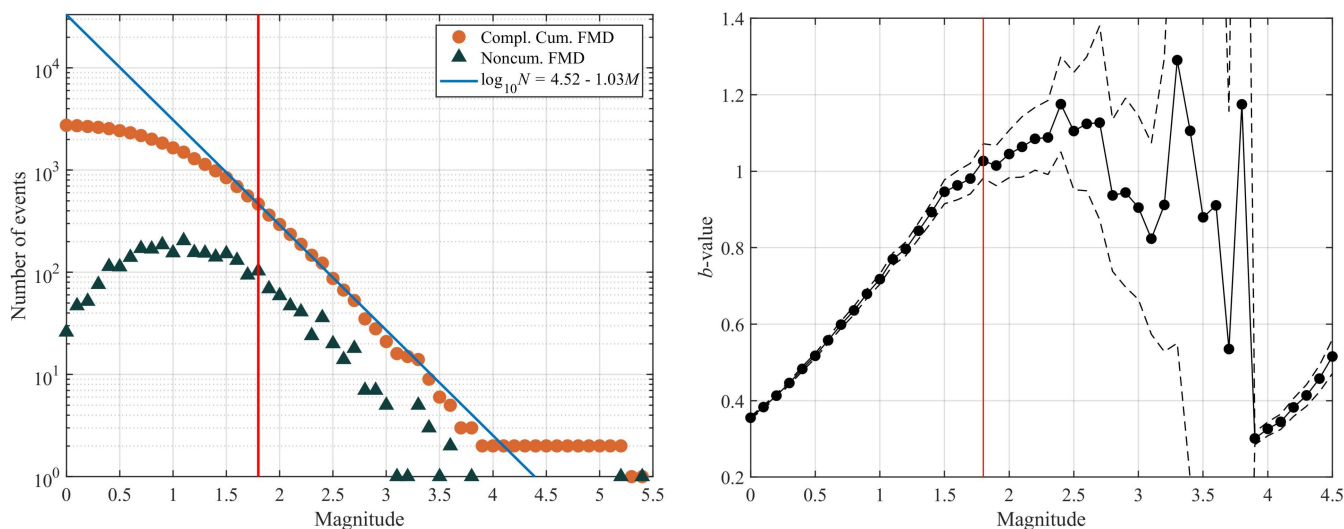
图 5. 过去一个月中国地震科学实验场地震活动性的 (左) 互补累积和非累积震级-频次分布及大于过去一个月的目录最小完整性震级 M_c (红竖线) 地震的古登堡-里克特 (GR) 关系拟合结果; (右) b 值随目录截止震级 M_c 变化的曲线, 其中细虚线表示 \pm 1\sigma 的标准差。
