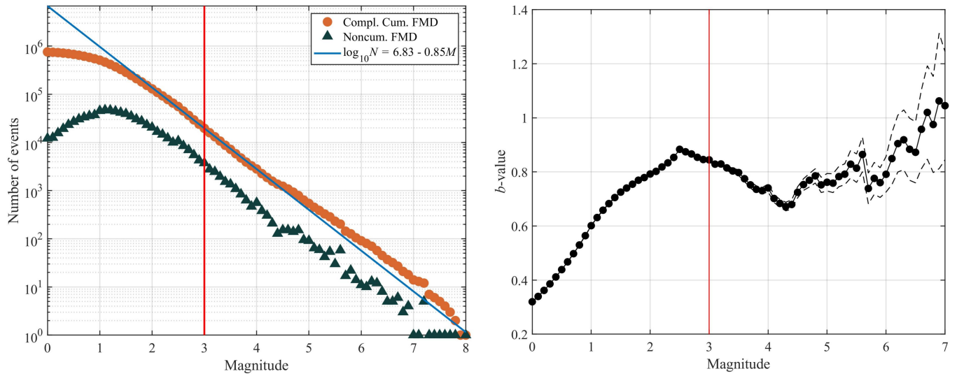
图 12. (左) 1970 年至今中国地震科学实验场内地震事件的互补累积和非累积震级-频次分布以及大于目录截止震级 M_{c0} = 3.0 (红线) 地震的古登堡-里克特 (GR) 关系拟合结果; (右) 相同地震目录 b 值随 M_{c0} 变化的曲线, 其中细虚线表示 \pm 1\sigma 的标准差。估计 b 值和拟合 GR 关系的方法详见 Li 等 (2024) 补充材料。
