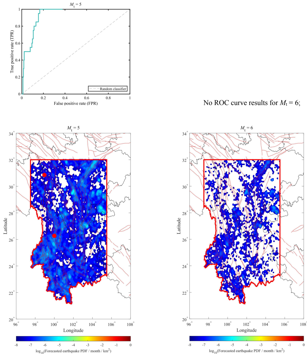
图 7. -同上。ROC 曲线是通过遍历所有预测的地震概率密度值并按降序计算出。对于每个概率密度阈值，计算真实发生地震所占网格的真阳性率 (TPR) 和假阳性率 (FPR)。在这种情况下，ROC 曲线是基于上个月度预测报告发布的预测地震 ( M \geq M_t ) 每平方公里概率密度分布所构建。这个过程涉及通过将预测的概率密度与该期间内实际发生的地震进行比较来评估预测模型的性能。
