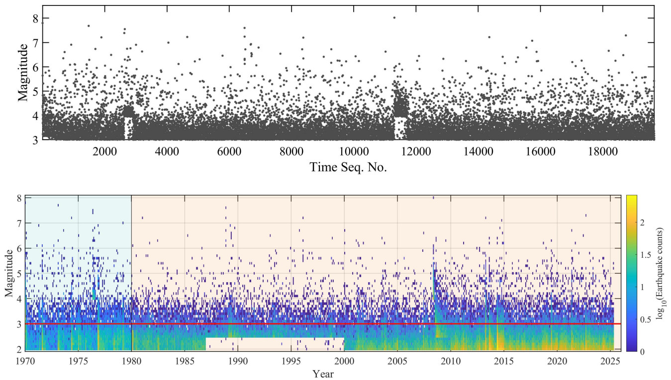
图 10. 中国地震科学实验场内自 1970 年以来地震活动性的 (上) 震级序号图及 (下) 每 0.1 个震级区间的每月地震数量。震级-时间序号图中的震级被添加了 [-0.05, 0.05] 均匀分布的随机误差。红线表示截止震级 M_{co} = 3.0 。浅红色和浅蓝色背景区域分别为主时段和辅助时段。截止震级 M_{co} 、主时段和辅助时段等参数均用于 ETAS 模型参数反演和预测模拟的构建。
