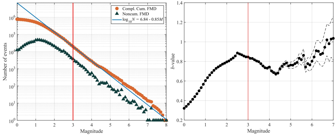
图 12. (左) 1970 年至今中国地震科学实验场内地震事件的互补累积和非累积震级-频次分布以及大于目录截止震级 M_{co} = 3.0 (红线) 地震的古登堡-里克特 (GR) 关系拟合结果; (右) 相同地震目录 b 值随 M_{co} 变化的曲线, 其中细虚线表示 \pm 1\sigma 的标准差。估计 b 值和拟合 GR 关系的方法详见 Li 等 (2025) 补充材料。
