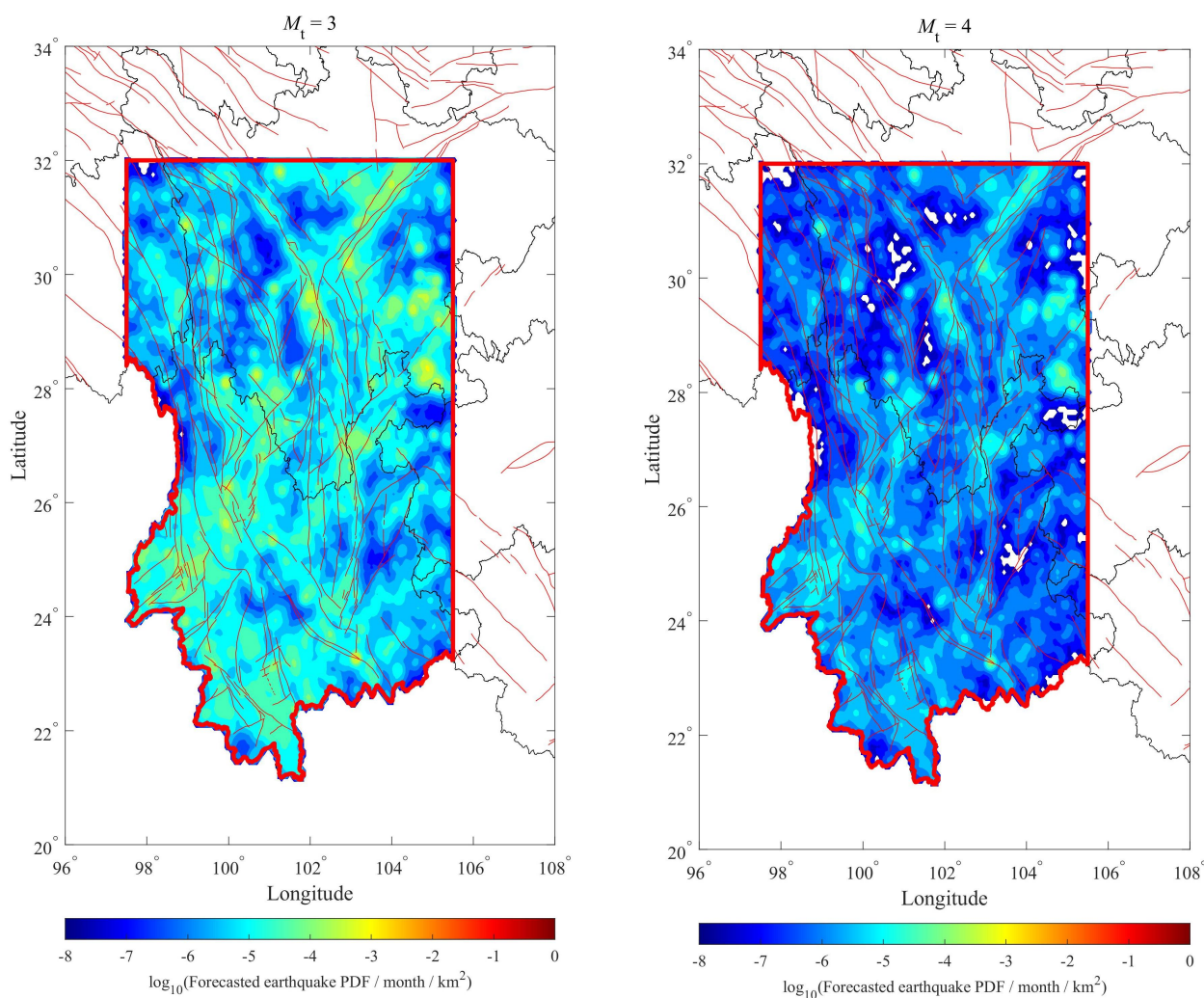
图 2. 未来一个月中国地震科学实验场内预测地震 ( M \geq M_t ) 每平方公里 ( \text{km}^2 ) 的概率密度分布 (PDF)。
