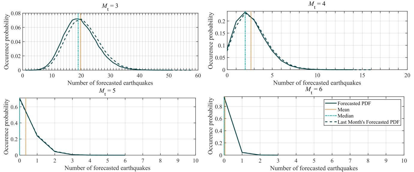
图 1. 未来一个月中国地震科学实验场 (川滇地区) 内不同震级范围 ( M \geq M_i ) 的地震数目预测概率。
