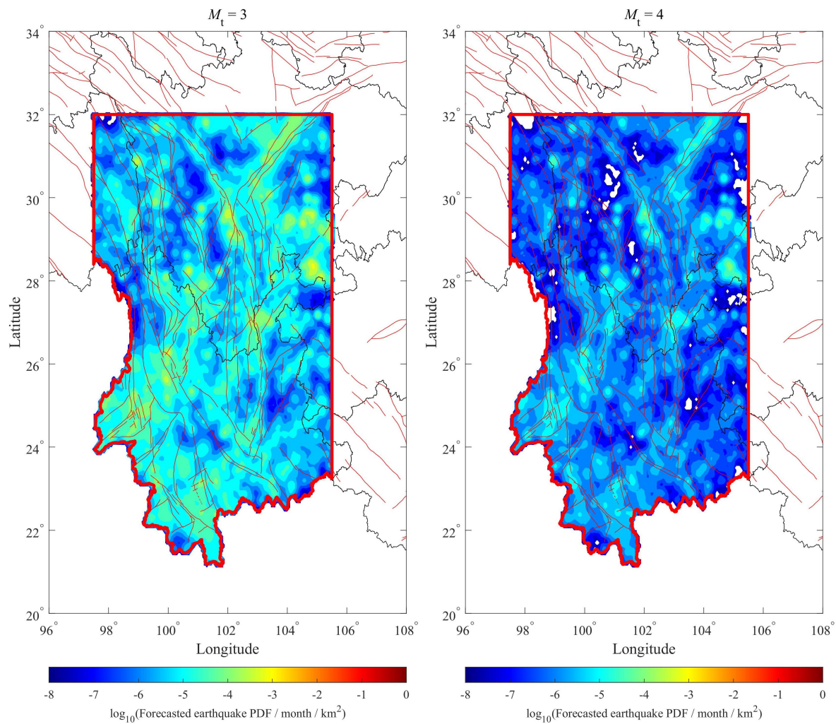
图 2. 未来一个月中国地震科学实验场内预测地震 ( M \geq M_i ) 每平方公里 ( \text{km}^2 ) 的概率密度分布 (PDF)。
