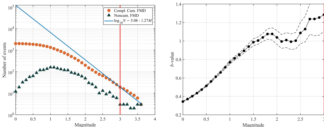
图 5. 过去一个月中国地震科学实验场地震活动性的（左）互补累积和密度震级-频次分布以及大于目录截止震级 M_{co} = 3.0 （红线）地震的古登堡-里克特（GR）关系拟合结果；（右） b 值随 M_{co} 变化的曲线，其中细虚线表示 \pm 1\sigma 的标准差。
